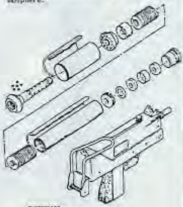
SUPPRESSOR M11 30MM PARA. C. M5ADP
